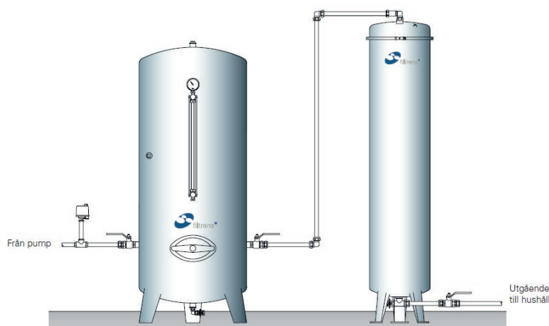
Installationsskiss
